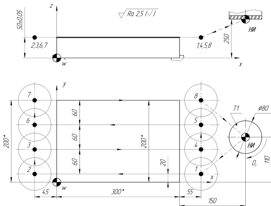
Рисунок 36. Эскиз расчетно-технологической карты
